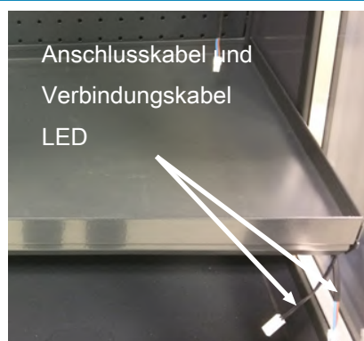
Abb. 11: Regalauslagen einhängen
