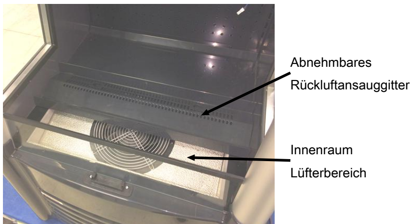
Abb. 16: abnehmbares Rückluftansauggitter
