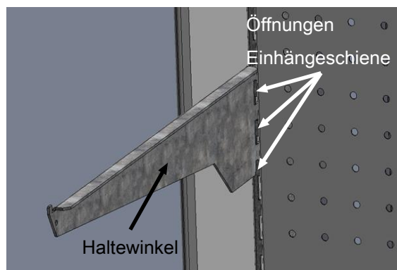
Abb. 10: Haltewinkel einhängen (ohne/mit LED-Balken)
